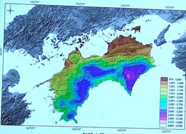
年降水量
